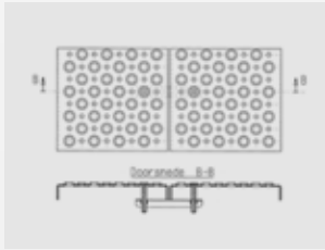
Couplingset AP Koppelset AP Doppelklemmsatz AP
