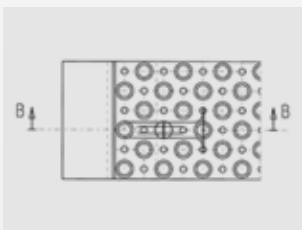
Fix clamping set AP Bevestigingsklemset AP Befestigungssatz AP
