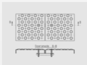
Couplingset AP Koppelset AP Doppelklemmsatz AP
